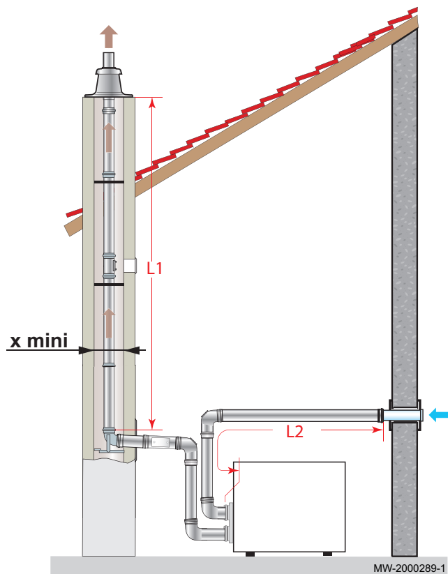
Fig.38 Raccordement de type C53 - Conduits air et fumées séparés avec adaptateur bi-flux (air comburant pris à l'extérieur)
