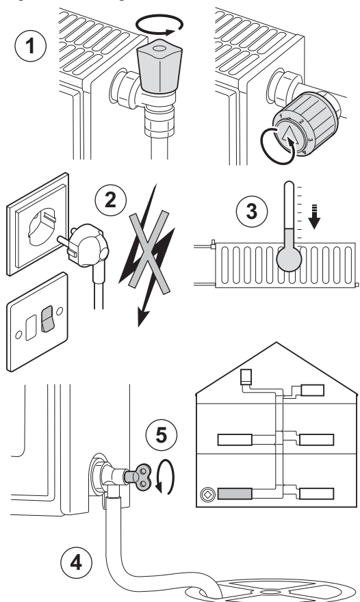
Fig.127 Vidange de l'installation
