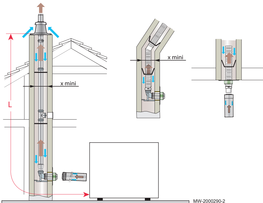
Fig.39 Raccordement de type C93 - Conduits concentriques en chaufferie ou conduits simples en cheminée (air comburant en contre-courant)
