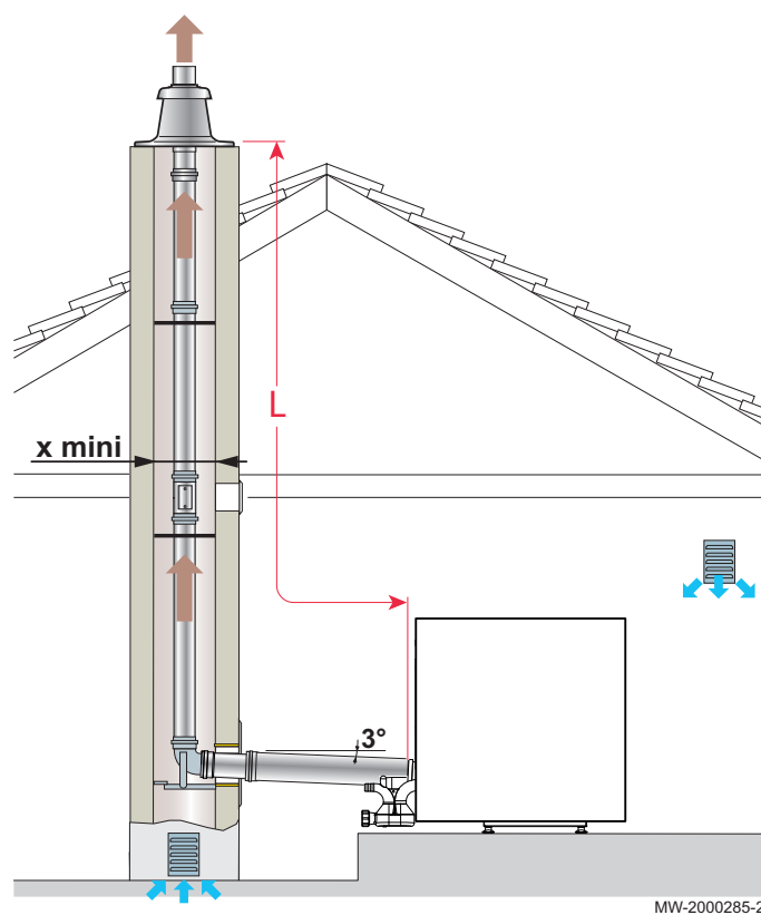
Fig.34 Raccordement de type B 23 et B 23P en rigide - Conduits de fumées (air comburant pris dans la chaufferie)
