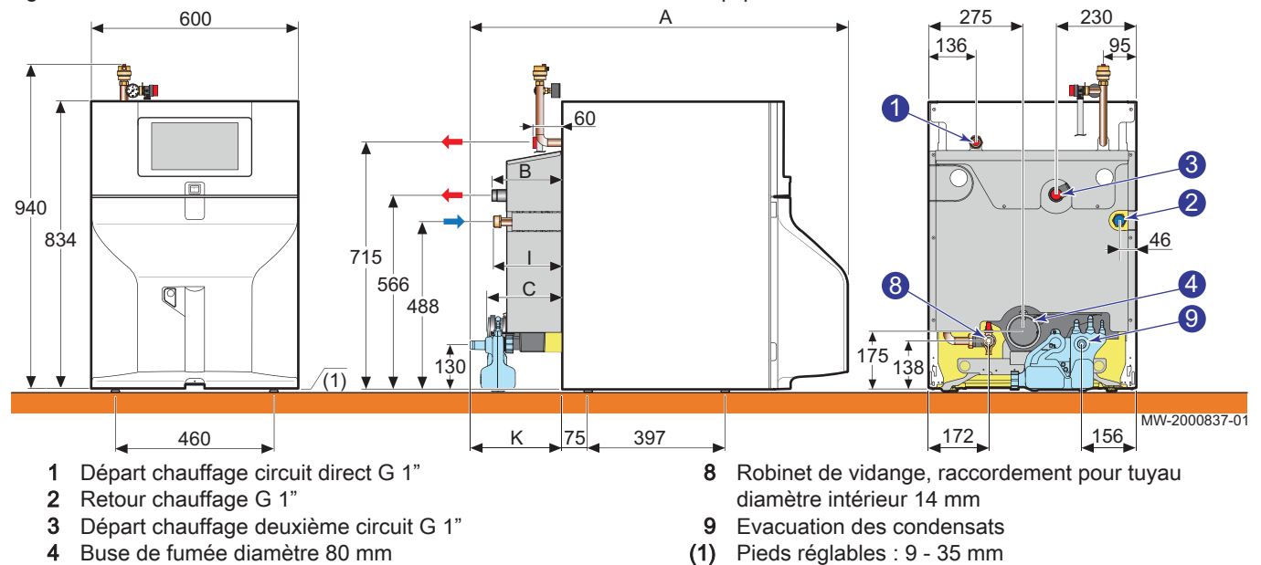
Fig.3 Chaudière HC 2-19 FF / HC 2-24 FF / HC 2-32 FF : avec kit équipement MY404
